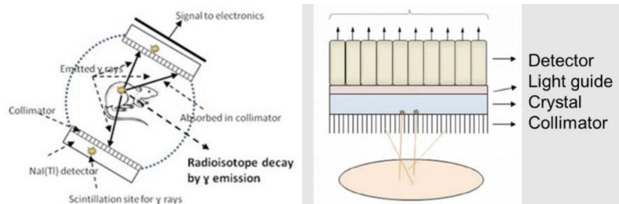
图 9-4 \gamma CUBE (SPECT) 原理示意图
