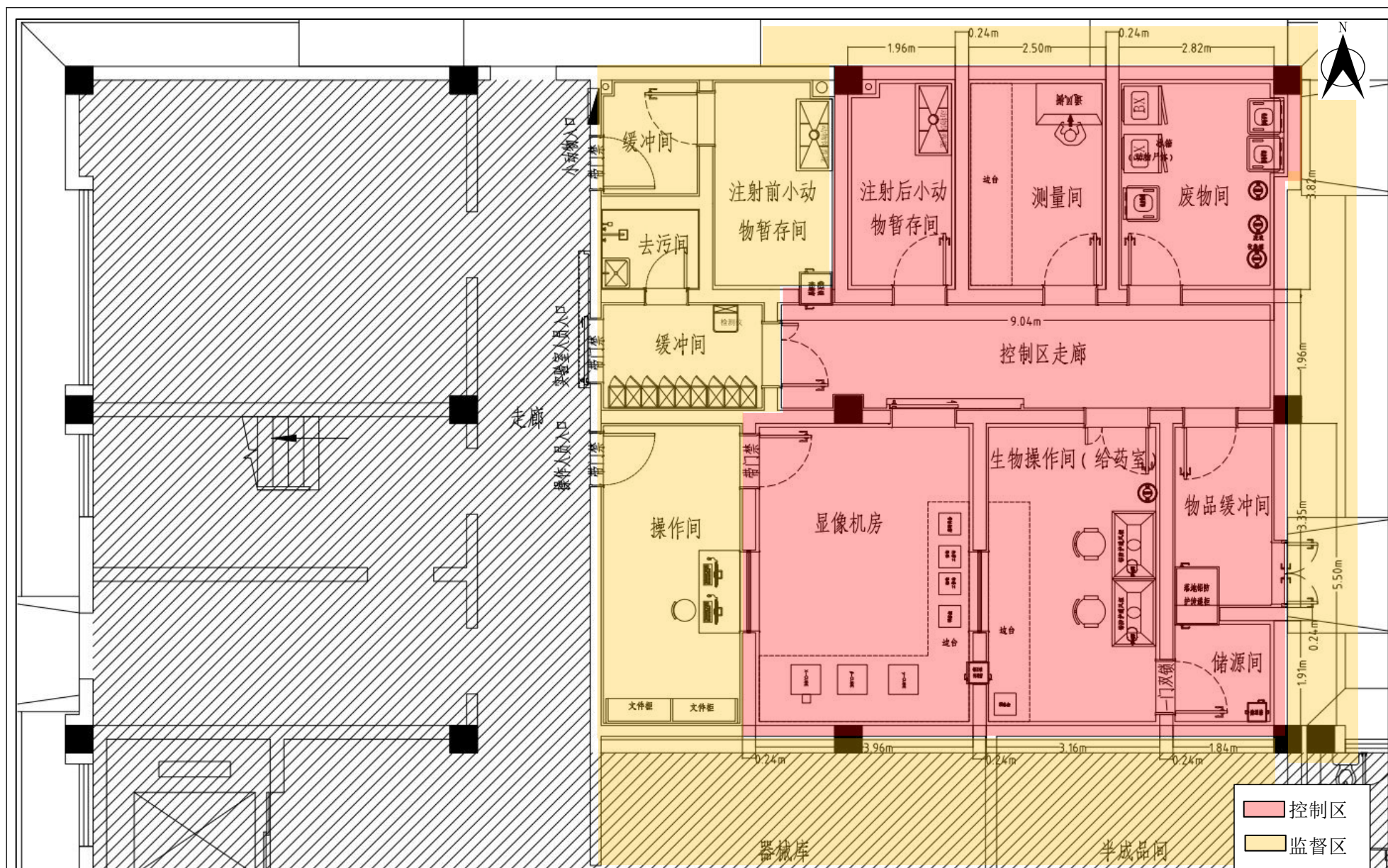
图 10-1 小动物实验室工作场所平面布置与分区示意图
