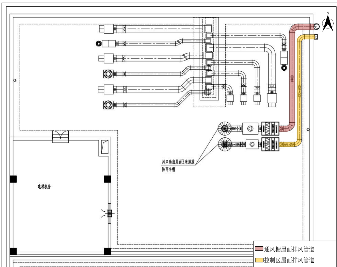
图 10-5 本项目小动物实验室屋面排风机平面图
