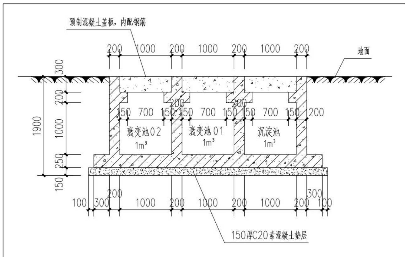
图 10-8 小动物实验室衰变池剖面图
