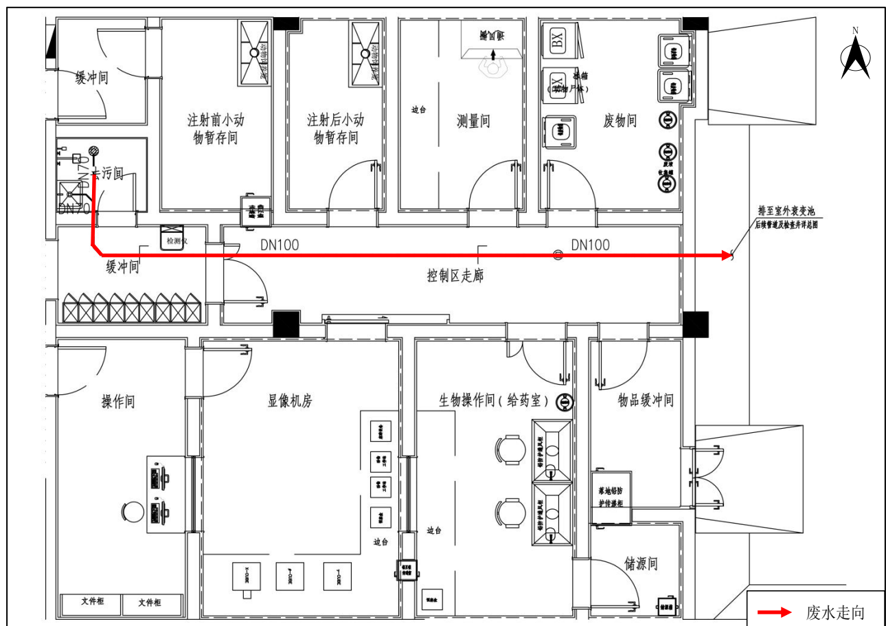
图 10-6 本项目小动物实验室排水水管平面分布及排水走向示意图
