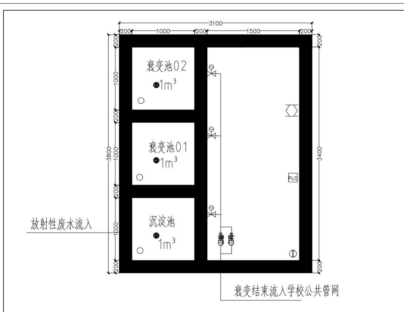
图 10-7 小动物实验室衰变池平面图
