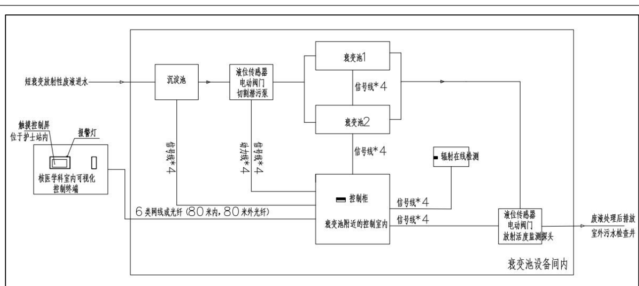
图 10-9 衰变池电气原理图
